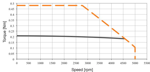
TETRA COMPACT 40 0,16 01
