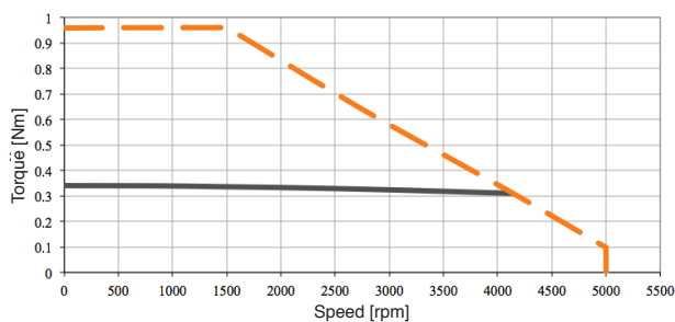
TETRA COMPACT 40 0,32 01
